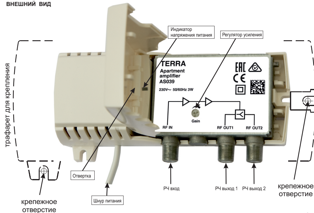
Рис.1. Внешний вид усилителя
